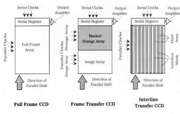
Figure 2 : Les différentes architectures de CCD
